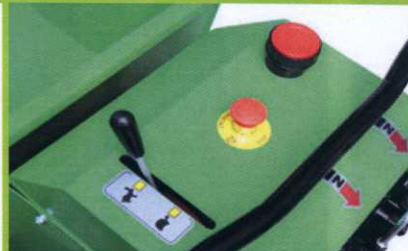
Leva comando doppia velocità versione TRS550 DV Double speed lever TRS550 DV model
